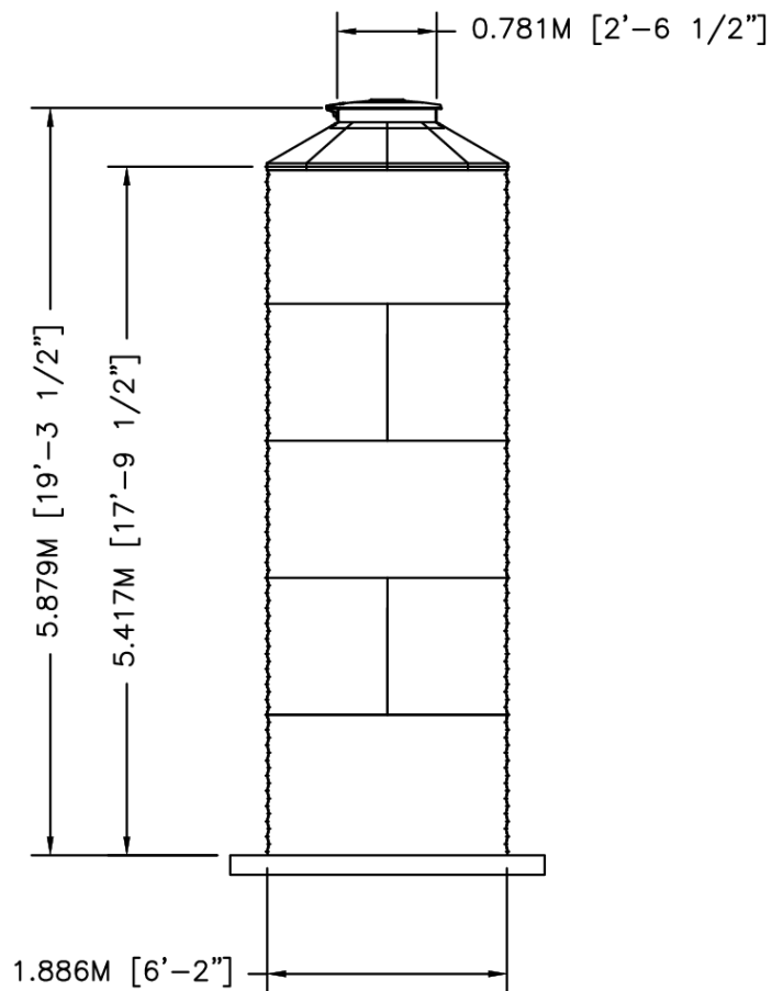
ELEVATION
